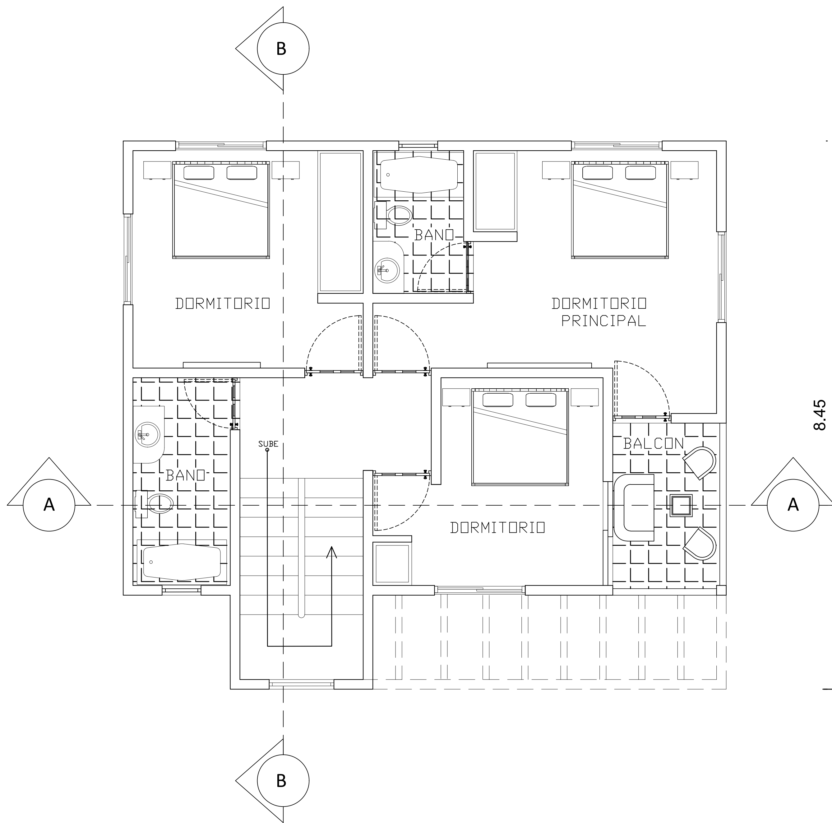
PLANTA ARQUITECTONICA AMUEBLADA SEGUNDO NIVEL
