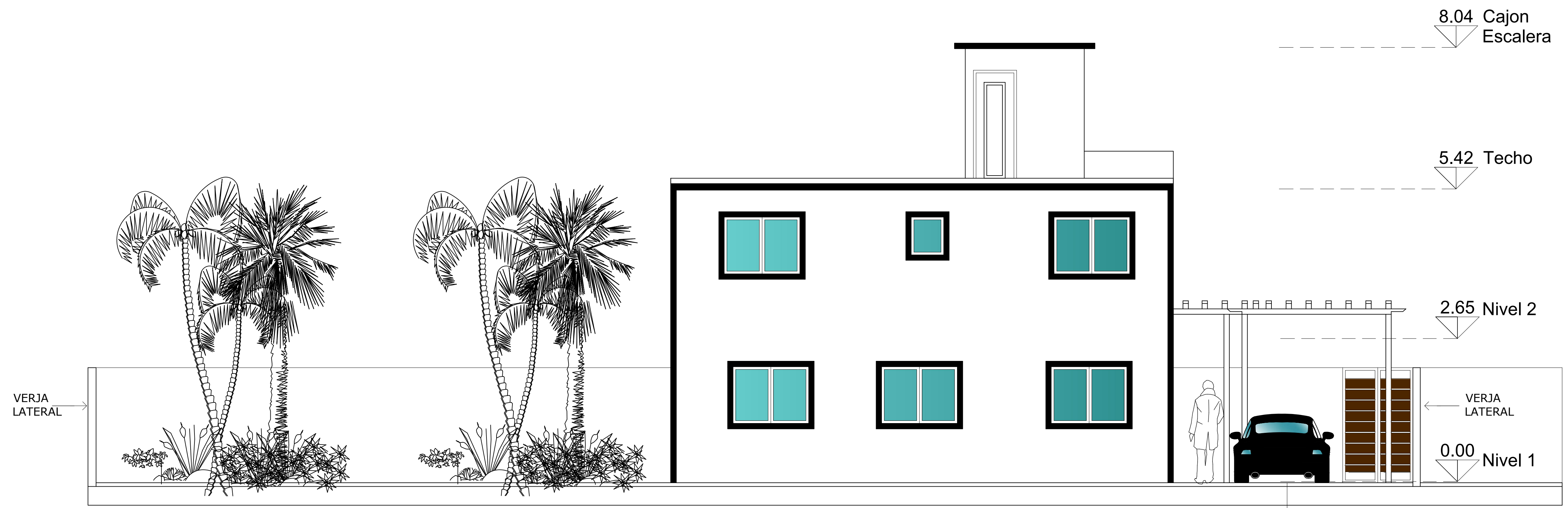
ELEVACION POSTERIOR
