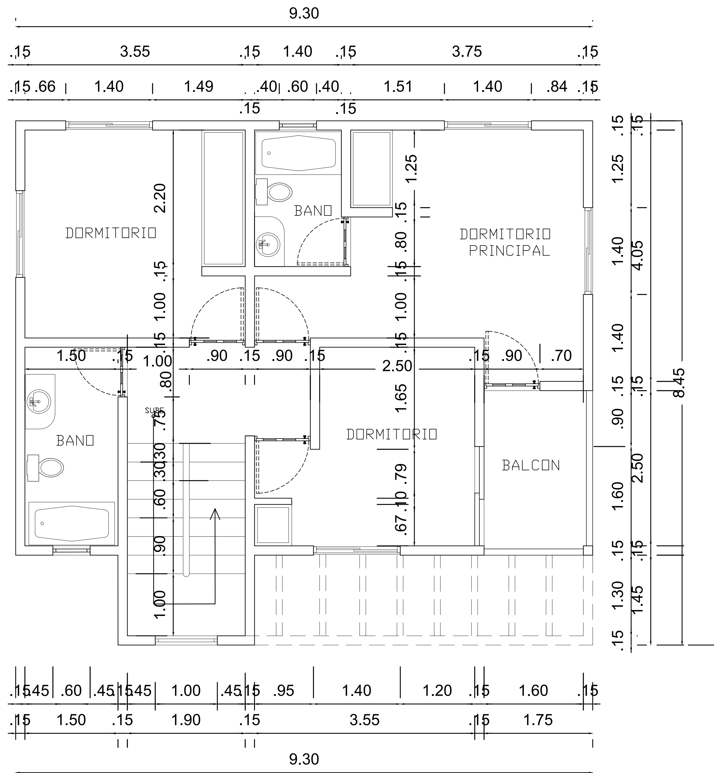
PLANTA ARQUITECTONICA DIMENSIONADA SEGUNDO NIVEL
