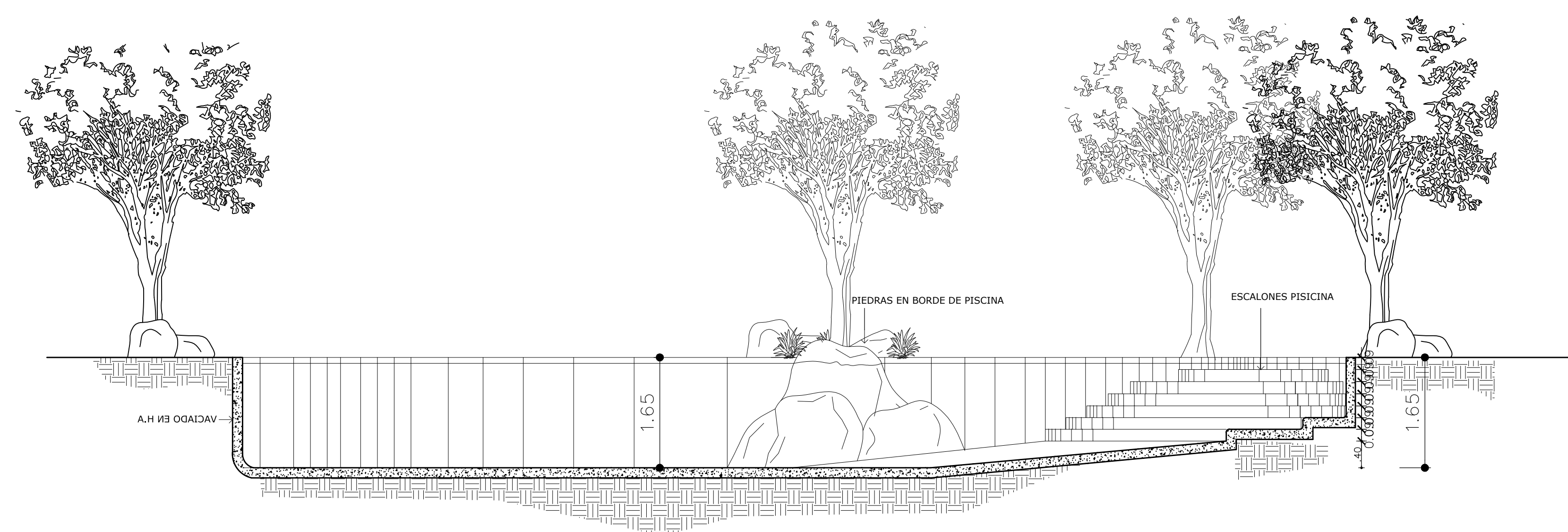
SECCION A-A
