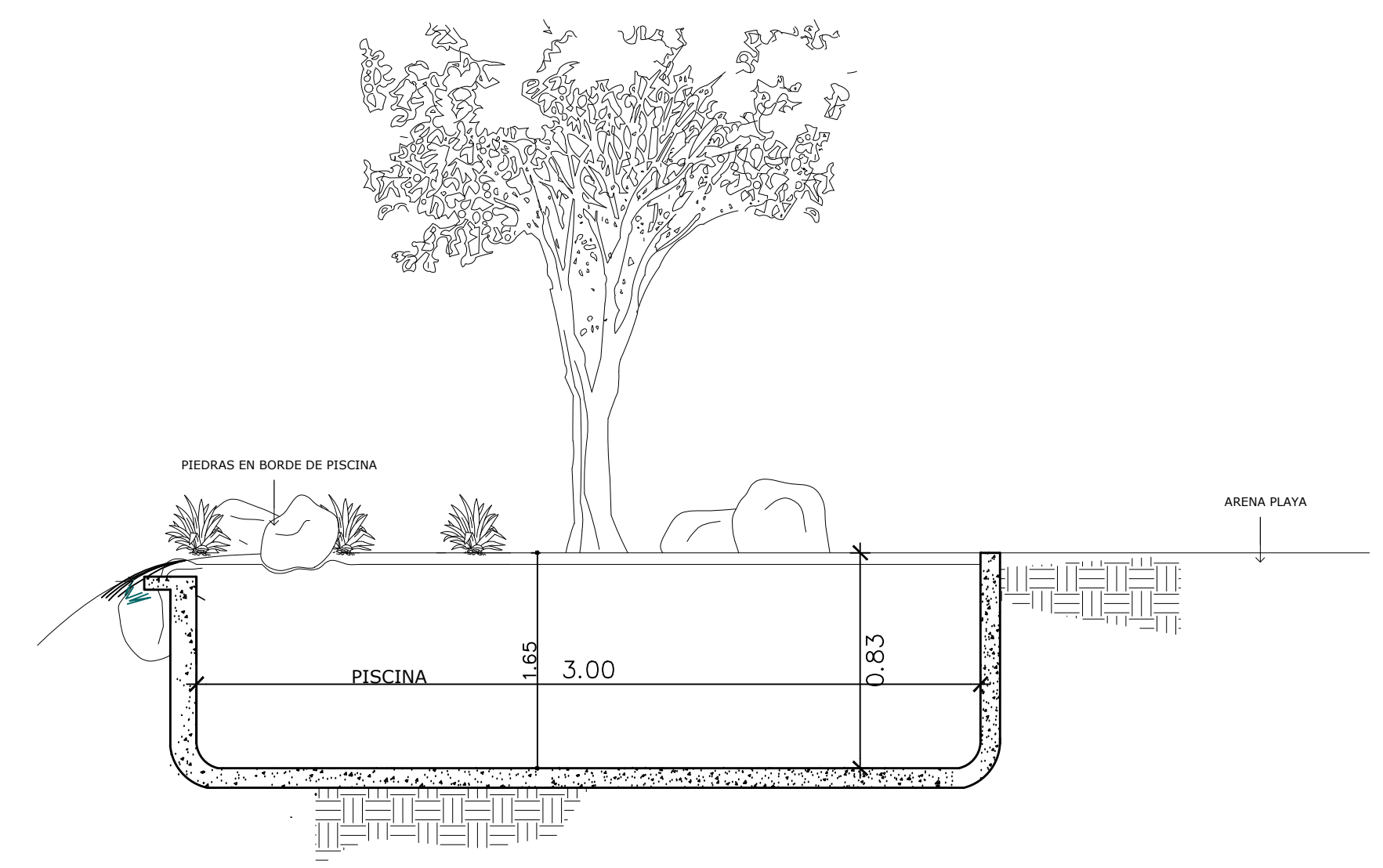
SECCION B-B
